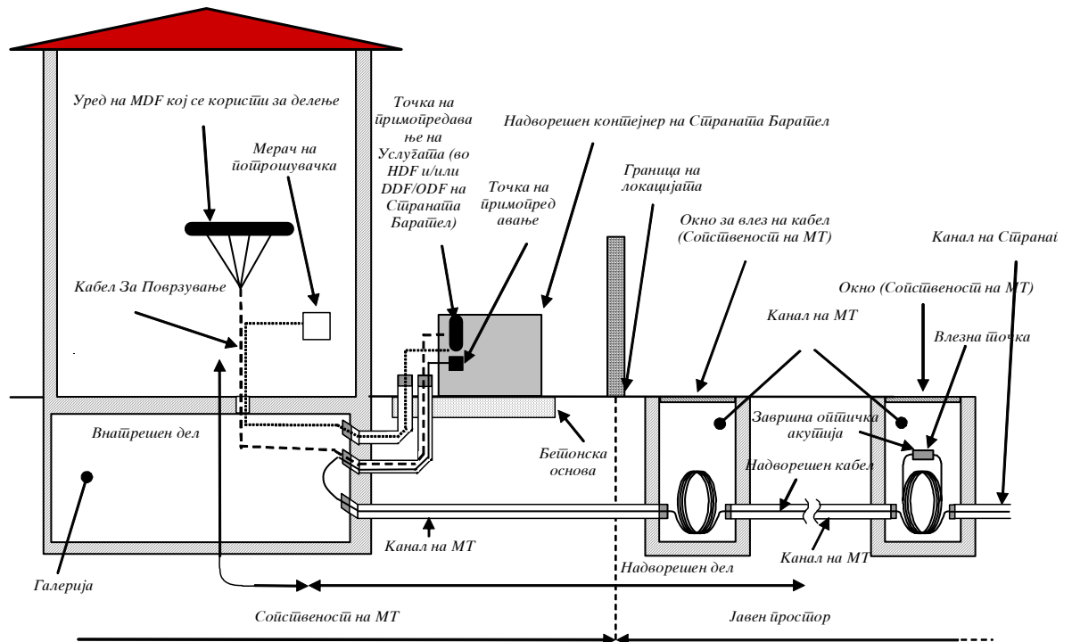
Слика 2 Шематски преглед на Оддалечена Колокација
